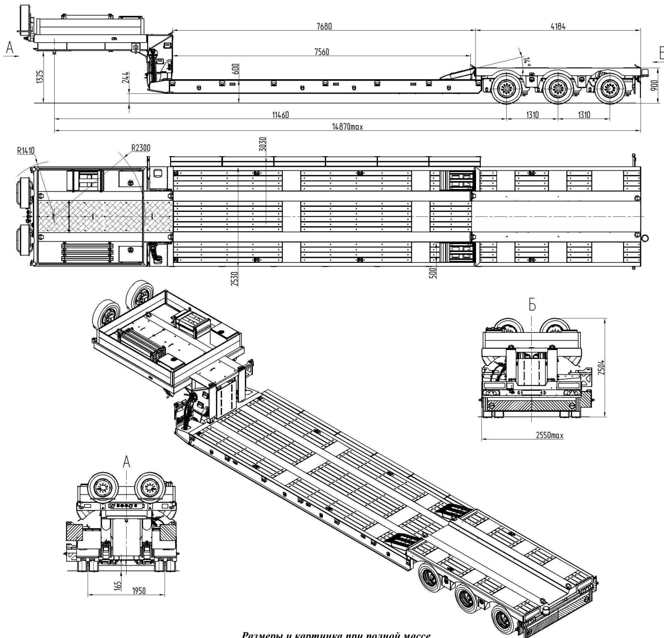
Размеры и картинка при полной массе
